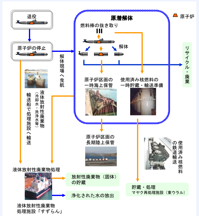
(図3) 原潜解体・処理のプロセス
